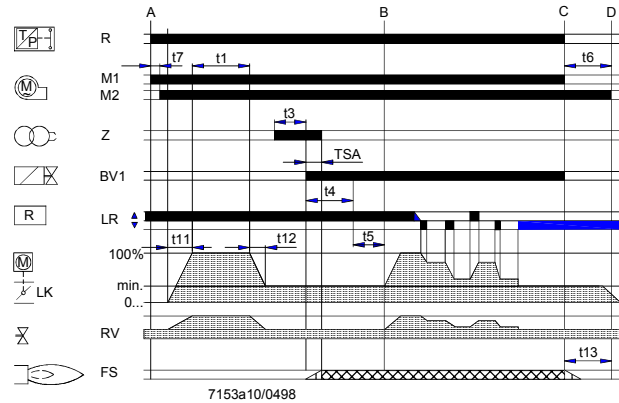
Einrohrbrenner, modulierend
