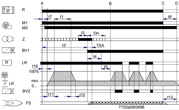
Einrohrbrenner, 2-stufig
